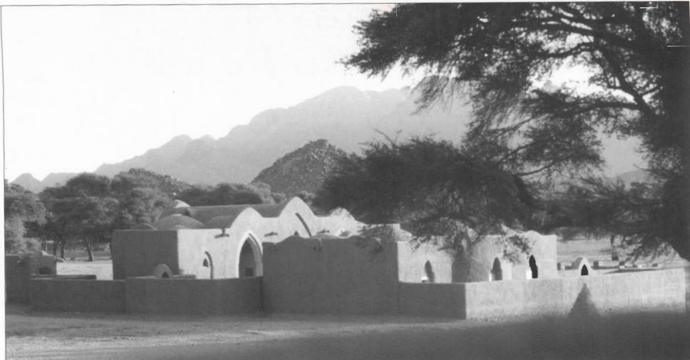
Figure 3 Voûtes et coupoles combinées pour des équipements confortables et attrayants
