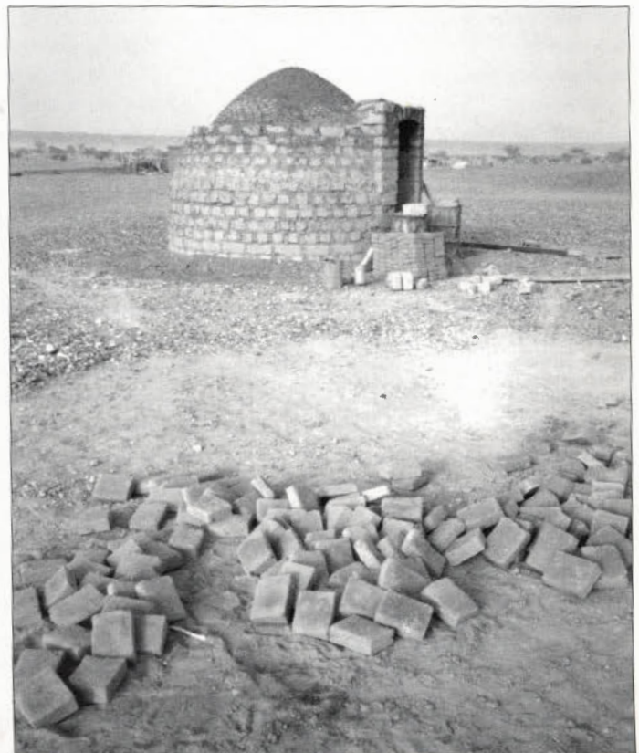
Figure 2 Structure ronde avec coupole – abri très économique, facile à construire
