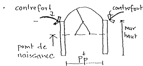
voûte surbaissée
