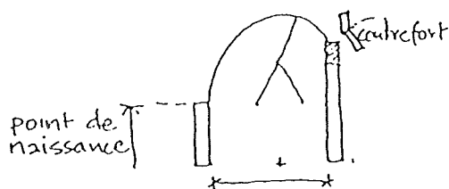
voûte excentrée
